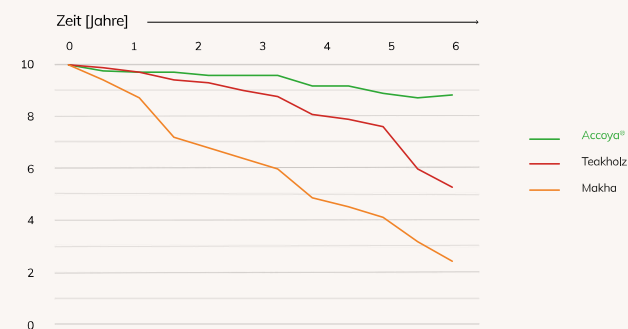
Termitenbefall [Zustandsindex]
