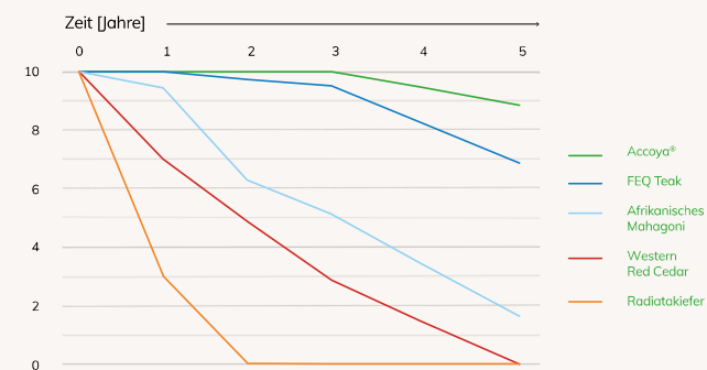
5 Jahre Zerfallsrate (E7 Bodenkontakt)
