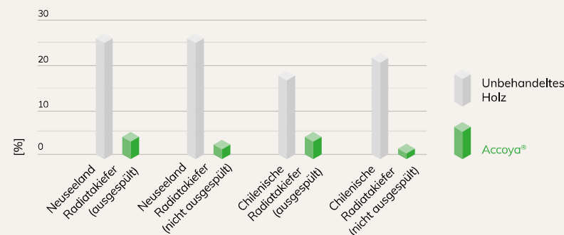
Gewichtsverlust beim LSU Termitentest
