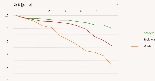
Zerfallsrate [Zustandsindex]
