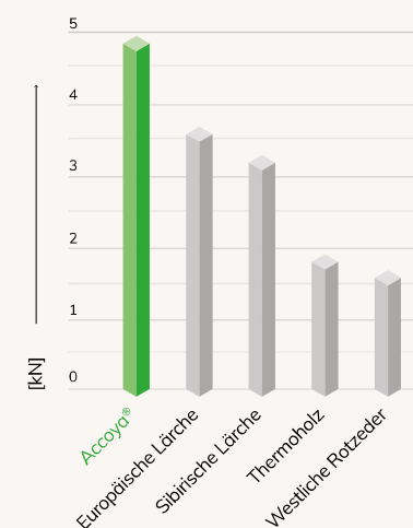
Mittlere Härtebelastung
