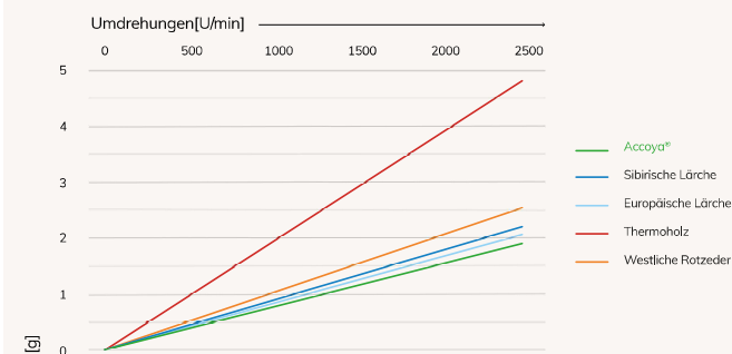
Gewichtsverlust durch Taber-Abrieb
