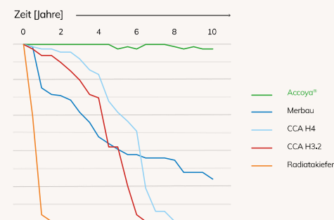
Zersetzungsdaten von Bodenpfählen [Zustandsindex]
