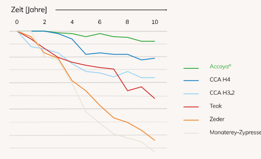
Zersetzungsdaten von Bodenpfählen [Zustandsindex]
